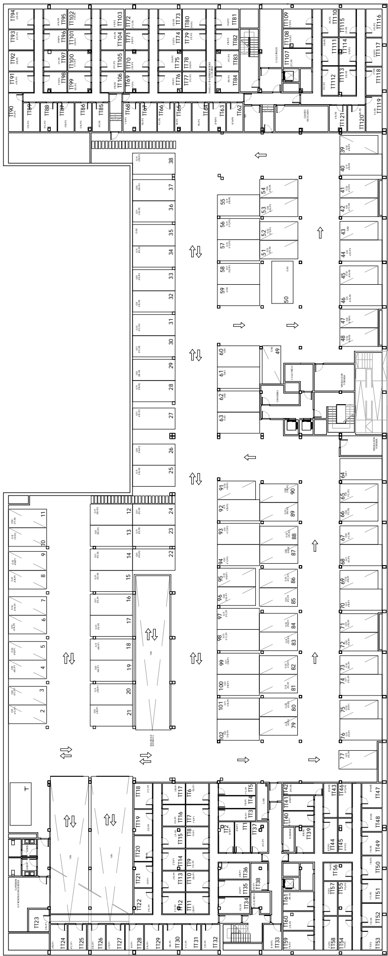
PLANTA SÓTANO 1
